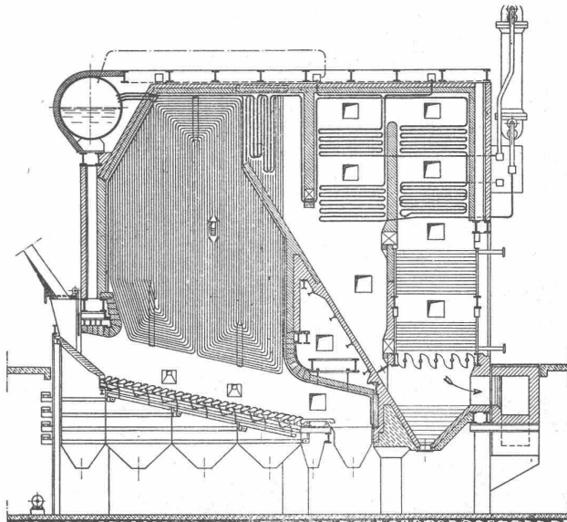
BUSS-La Mont -Dampferzeuger für 32/40 t/h, 50 at, 460° C, aus- gerüstet mit BUSS-ÜBERSCHUBROST .
