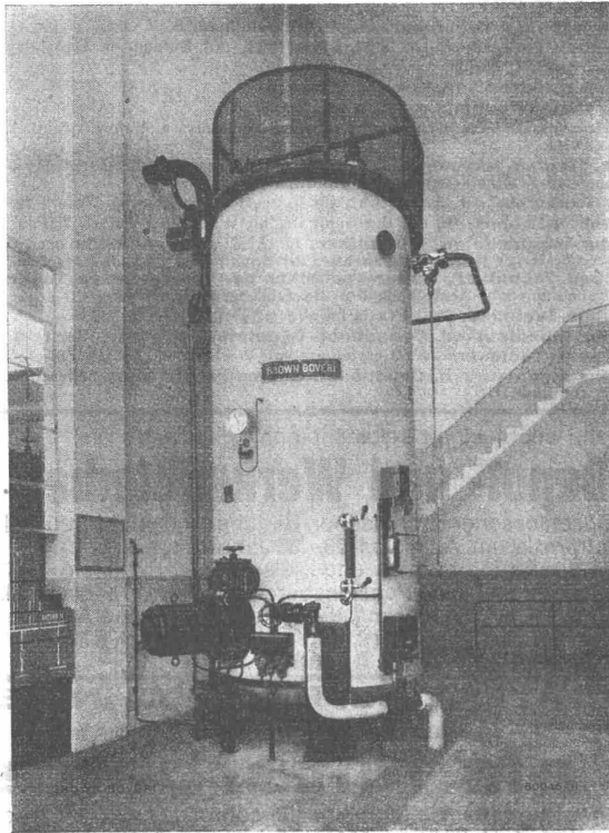
Elektrodampfkessel, 4500 kW, 16 000 V, 10 kg/cm 2
