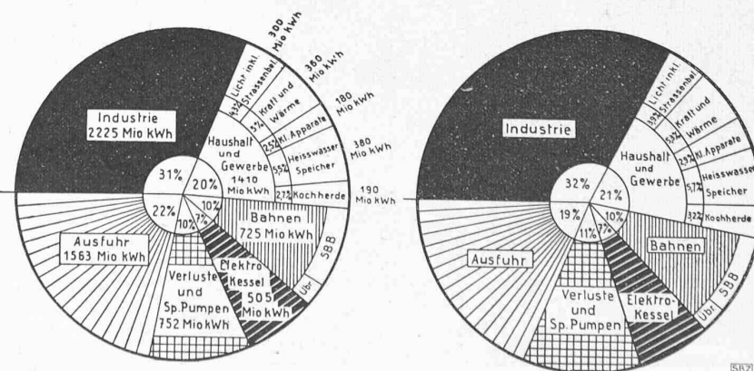
Abb. 7. Verwendungsarten der durch alle schweizerischen Wasserkraftwerke erzeugten Energie, links für 1938/39, rechts für 1941/42
