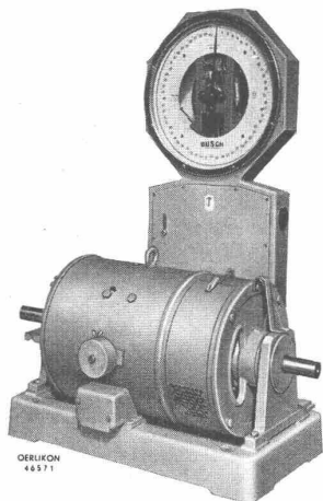
Moderne Leistungswaage Typ 57, mit automatischer Präzisionsschnellwaage, als Generator arbeitend: 3 ... 45 kW als Motor arbeitend: 3,5 ... 55 kW Drehzahlbereich: 400 ... 4000 U/min
