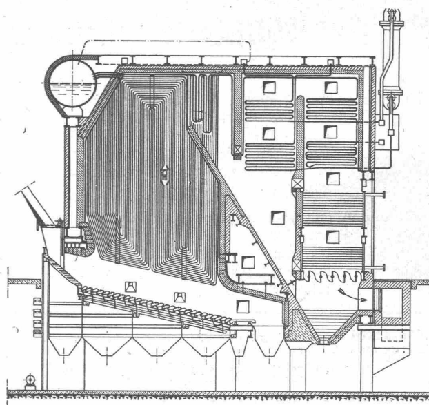
BUSS-La Mont-Dampferzeuger für 32/40 t/h, 50 at, 460° C, ausgerüstet mit BUSS-Ueberschubrost.
