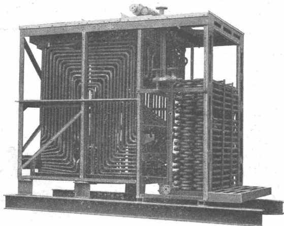
BUSS-La Mont-Heisswassererzeuger für 50 000 WE/h, 205° C.
