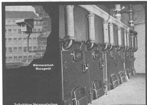
Selbsttätige Heizregelanlage
