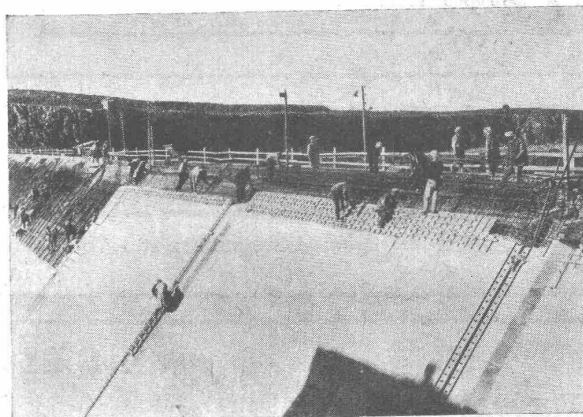
Staumauer Bakhadda (Nordafrika) Staumauer-Verkleidung ausgeführt mittels Plastiment-Beton.
