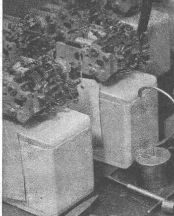
HEBDREHWÄHLER MIT KON- TAKTBANK UND RELAISSATZ
