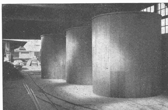
Innere Schalungen für Grünfuttersilos (Häring & Cie., A.-G., Frenkendorf)
