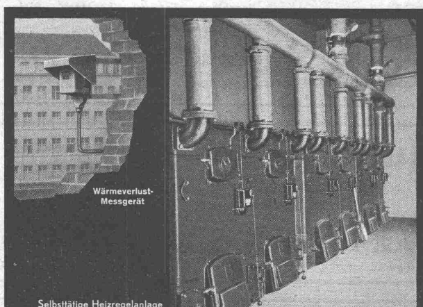
Selbsttätige Heizregelanlage
