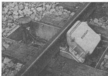
Impulsgeber für Achszählung
