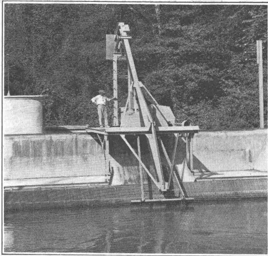
Vollautomatische Rechenreinigungsmaschine
