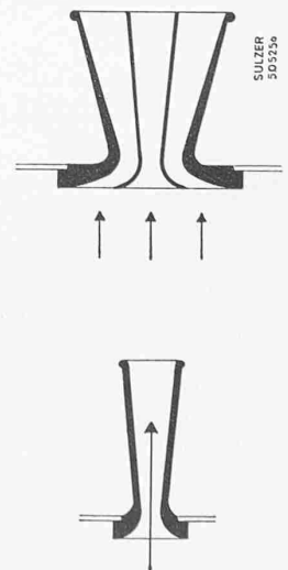
Abb. 10. Einfache und unterteilte Venturidüse
