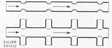
Abb. 8. Kondensatorkette nach A. Kauffmann und U. Schmidt. — C Kondensator, D Drossel
