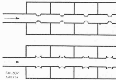
Abb. 7. Auspufftopf als Tiefpassfilter
