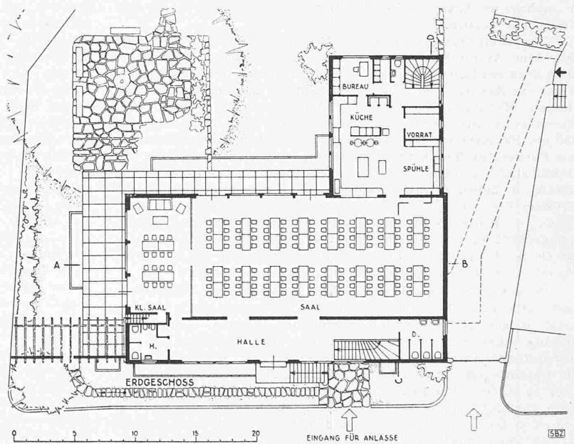
Abb. 8. Grundriss vom Saalgeschoss mit Küchenflügel. — 1 : 400
