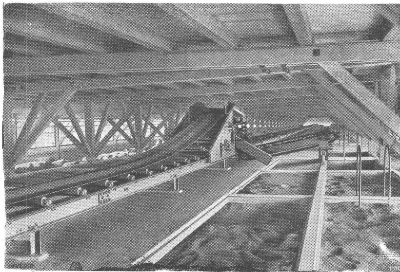
Transportanlage für loses und gesacktes Getreide in einem schweizerischen Lagerhaus
