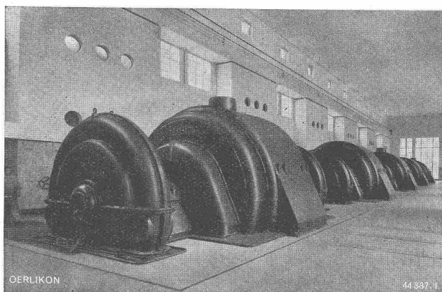
Zentrale La Dixence (Wallis) — grösstes „Hochdruck-Kraftwerk Europas“ — ausgerüstet mit fünf Oerlikon-Generatoren von je 37 500 kVA und einem Oerlikon-Hilfsgenerator von 7000 kVA. Installierte Leistung total 194 500 kVA
