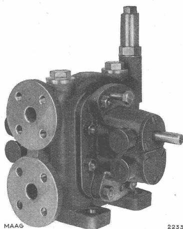
Von Dieselmotor angetriebene, automatisch umsteuerbare MAAG-Zahnradpumpe mit Aussenlagern zur Förderung von Süss- und Salzwasser.
