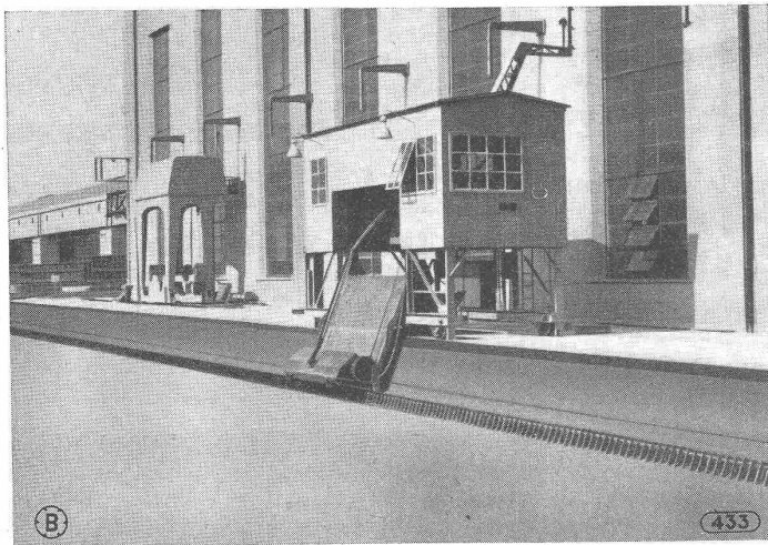
Rechenreinigungsmaschine Klingnau
