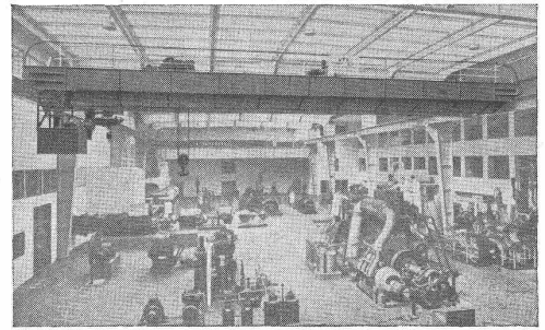
Maschinen-Laboratorium der E.T.H. Zürich. Geliefert: 3-Motoren-Lautkran für 10 T. mit Hilfskatze 2 T. Tragkraft.
