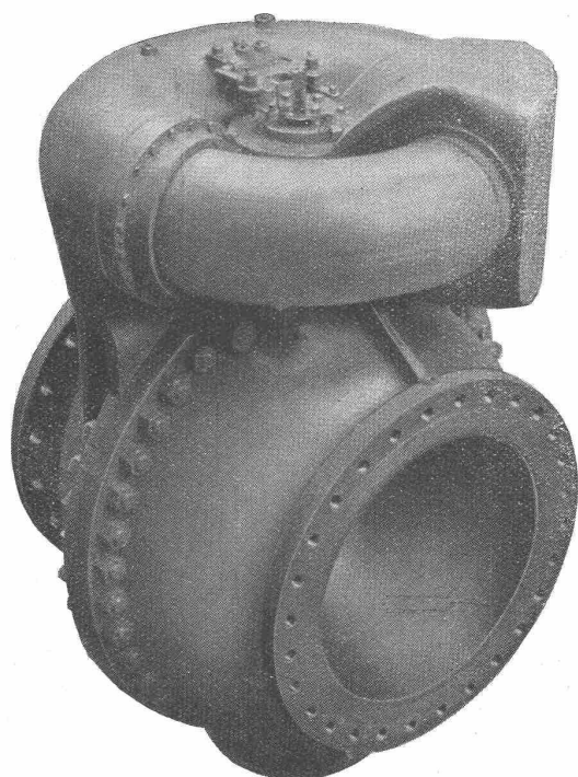
Drehschieber als Turbinenabschlussorgan, 1000 mm NW, 35 at Druck.
