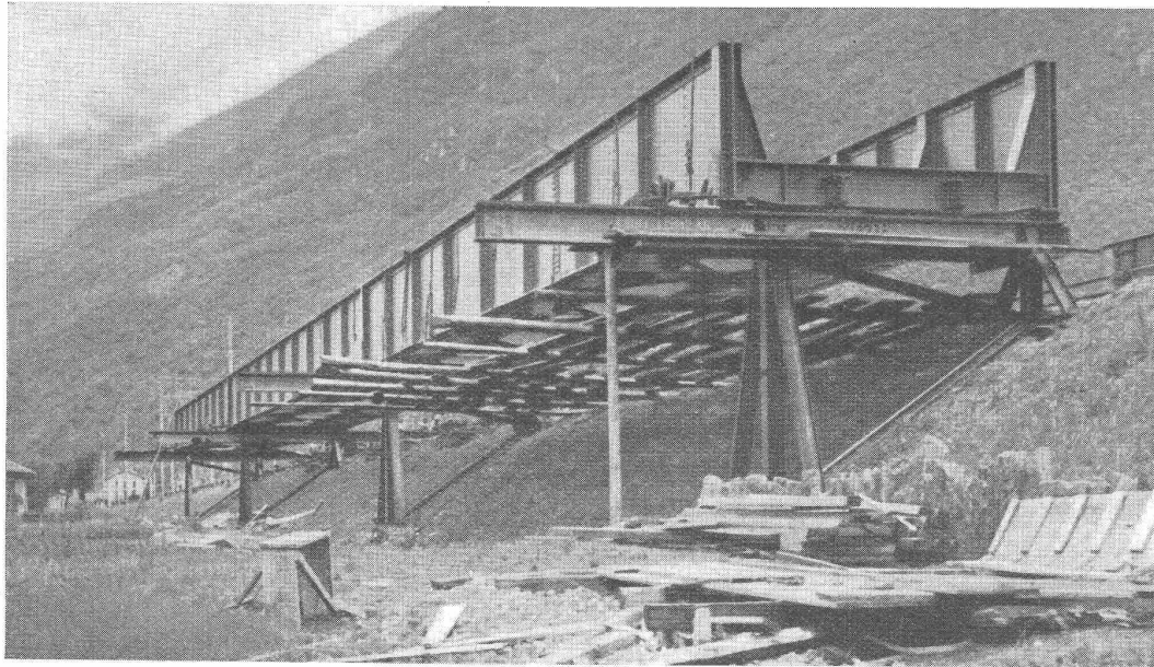
SBB eingeleisige Bahnbrücke über die Moesa, Tessin
