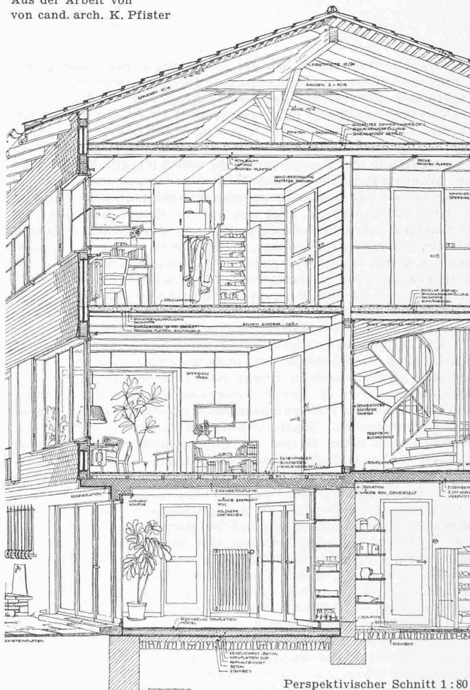
Perspektivischer Schnitt 1:80
