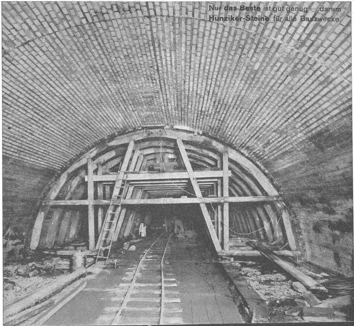
BOMMERSTEIN-TUNNEL der S.B.B. am Walensee Verkleidung mit Hunziker-Spezialsteinen
