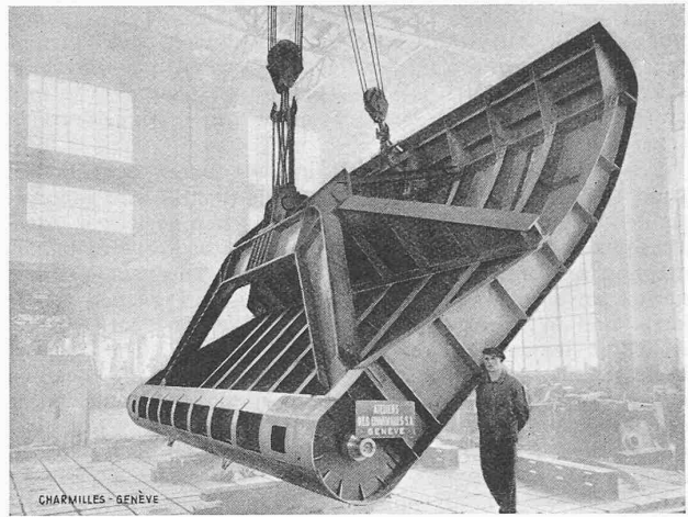
Abb. 2. Eine Stauklappe im Werk des Herstellers
