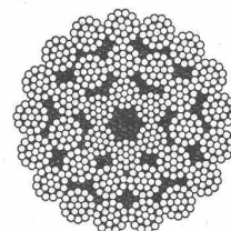
torsionsfreie Litzen-spiral- konstruktion mit Faser- stoffeinlagen
