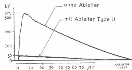
Verlauf einer Ueberspannungswelle
