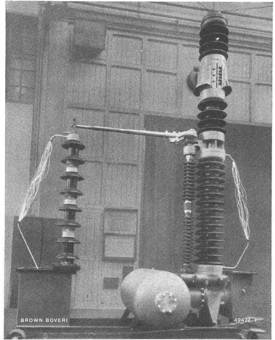
150 - kV - Druckluftschaltapparat Prüfung mit Stossspannung
