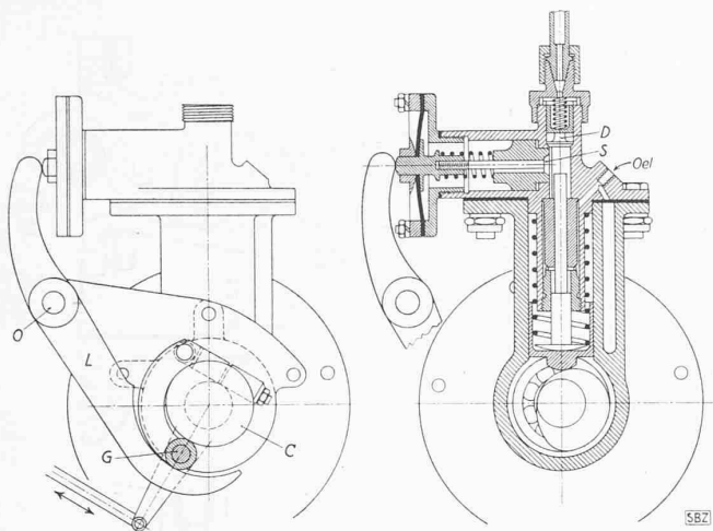
Abb. 4. Benzineinspritzpumpe von Lorraine. Rechts Schnitt, Links Mengen-Regulier-Vorrichtung. D Druckventil, S Saugventil, C Einspritz-Mengenregulirnocken, G Verstellrolle am Hebel L, O Drehpunkt des Hebels L
