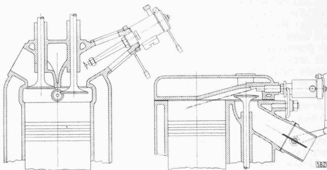
Abb. 6. Die Anordnung der elektromagnetischen Einspritzdüse von Caproni a) Einbau bei obengesteuertem Motor. b) Einbau bei Seitenventilen
