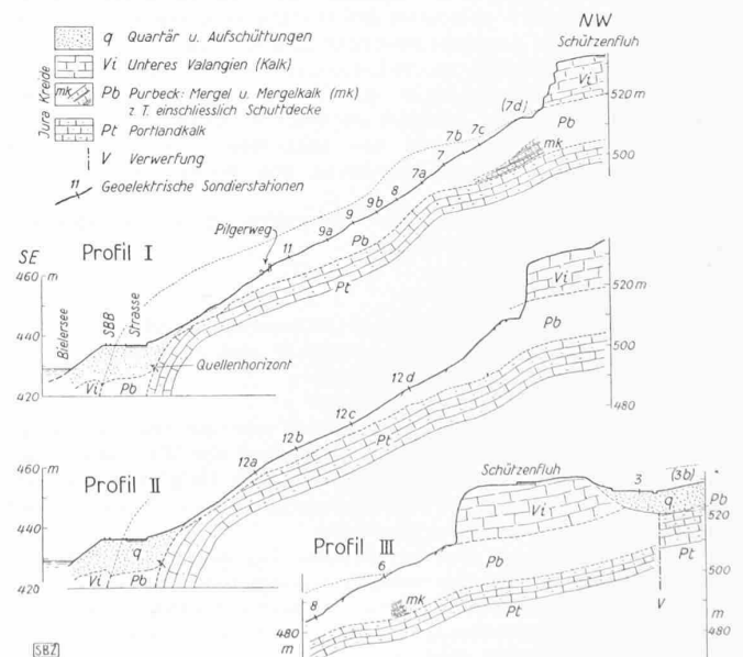
Abb. 5. Geologisches Profil gemäss geoelektr. Sondierung. — 1 : 2500
