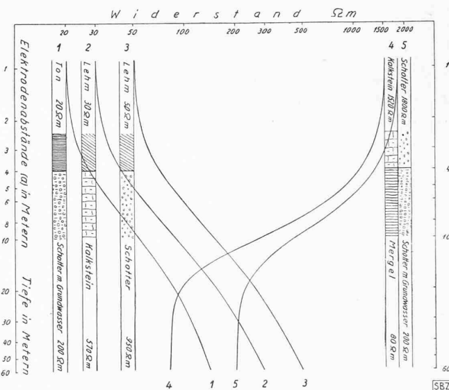
Abb. 1. Geoelektr. Sondierung, Zweischichtenproblem, Schichtgrenze 4 m
