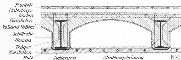
Abb. 39. Anordnung der Sulzer-Deckenheizung in den Obergeschossen
