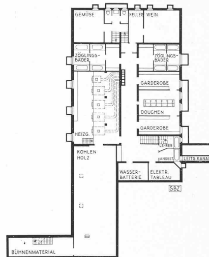
Abb. 11. Kellergrundriss 1 : 500
