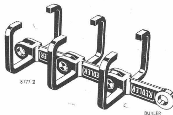
Kettenglieder
