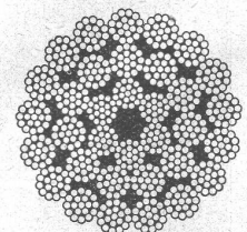
torsionsfreie Litzen-spiral- konstruktion mit Faser- stoffeinlagen
