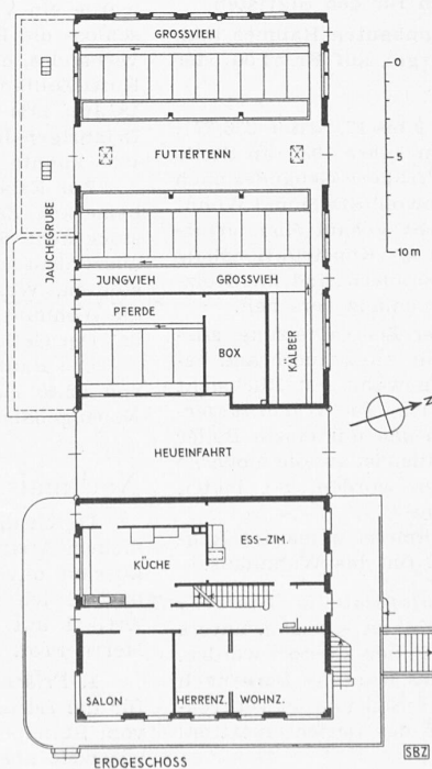
Abb. 9 bis 11. Grundrisse 1:400
