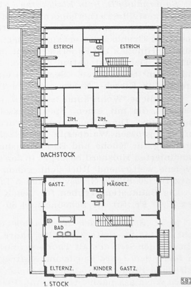
Abb. 9 bis 11. Grundrisse 1:400
