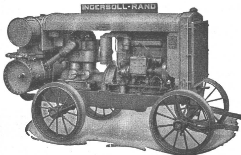
Rohölkompresseur 20/26 PS.
