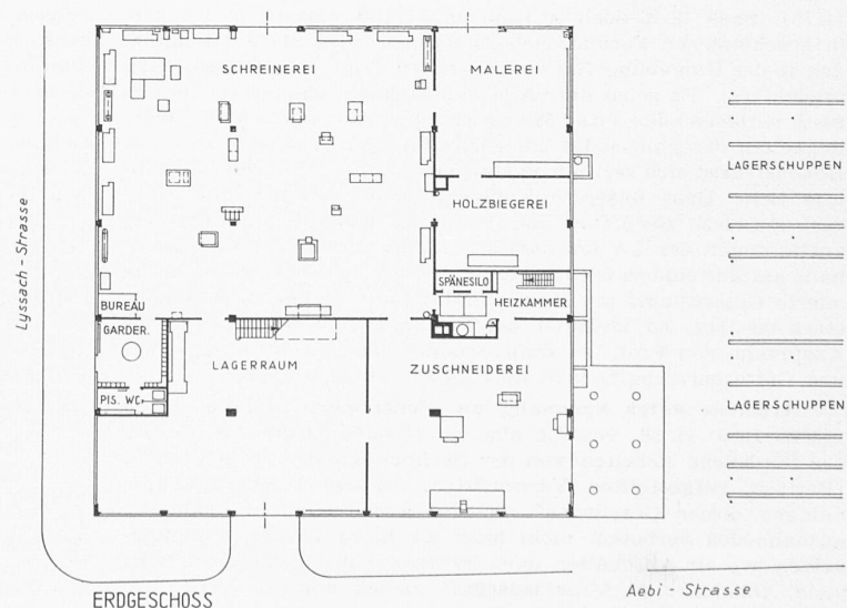
Abb. 1 und 2. Schreinerei- und Heizungsgebäude der Maschinenfabrik Aebi & Cie. in Burgdorf. — Masstab 1 : 500
