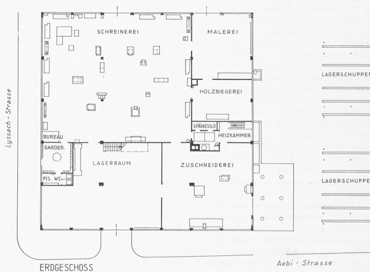
Abb. 1 und 2. Schreinerei- und Heizungsgebäude der Maschinenfabrik Aebi &amp; Cie. in Burgdorf. — Masstab 1:500
