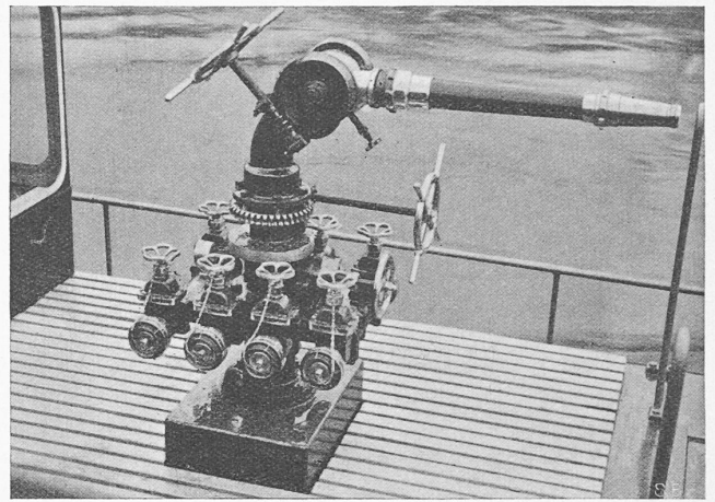
Abb. 3. Wasserkanne und Schlauchanschluss-Batterie
