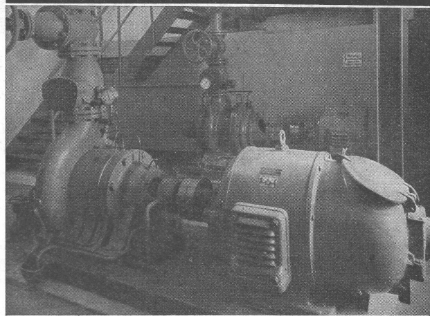
Hochdruck-Zentrifugpumpe 115 P.S.
