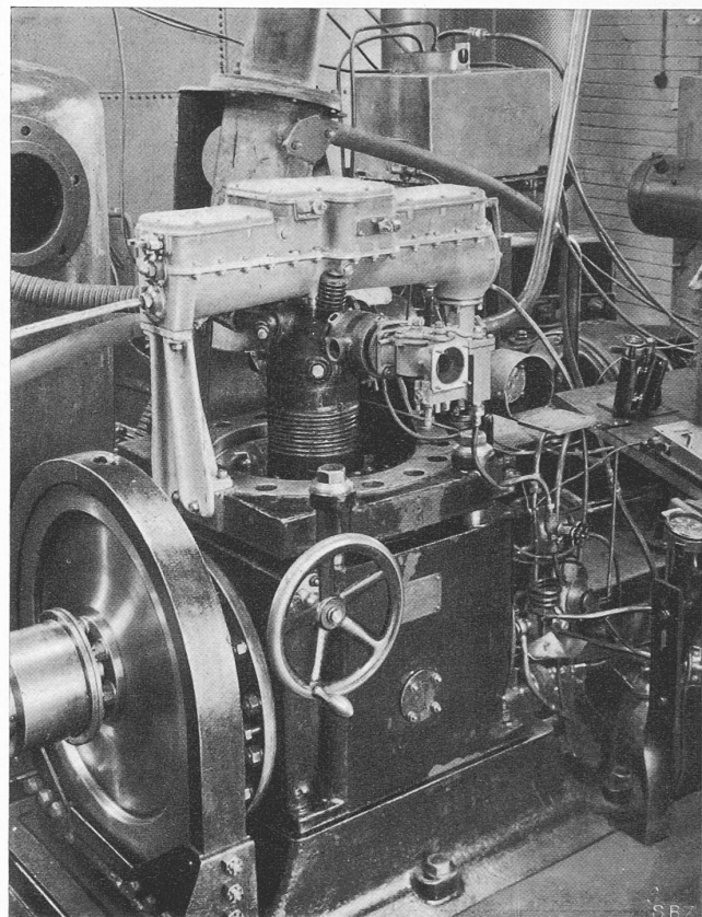
Abb. 8. Einzyylinder-Versuchstand der DVL mit BMW-Flugmotor-Zylinder von 3,82 l Hubvolumen
