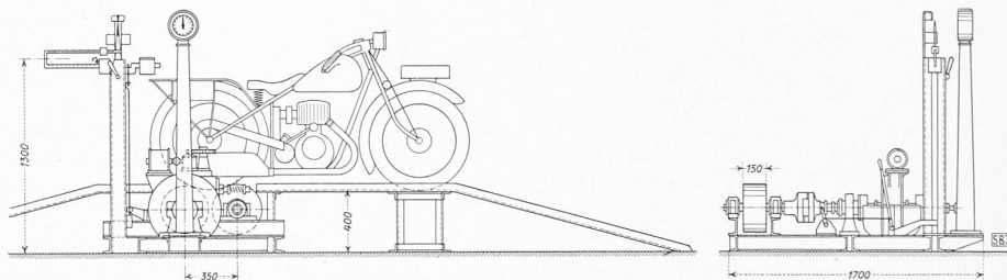
Abb. 7. Motorradrollstand Schenck, Darmstadt, mit 14,5 PS-Einzyylinder-Motosacoche-Rad. — 1:50
