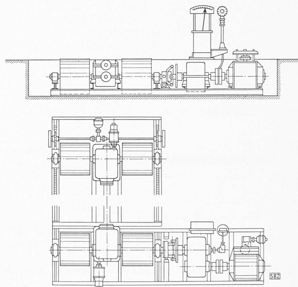
Abb. 5. Automobil-Rollfeld von Schenck, Darmstadt. — 1:100
