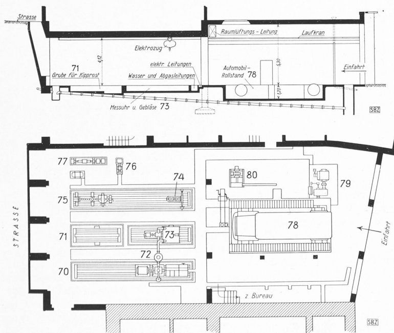
Abb. 1 u. 2. Grundriss und Schnitt des Leichtmotoren-Laboratoriums der E. T. H. — 1:300. Legende (vergl. den Gesamtgrundriss in Bd. 106, S. 144): 70 Aufspannrost, 71 Kipprost, 72 Einzyylinder-Prüfstand der DVL, 73 Luftmengenmessuhr, 74 Saurer Lastwagenmotor mit Prony-Zaum, 75 Argus Flugmotor mit Junkers-Wasserwirbelbremse, 76 Pleuelwaage, 77 Auswuchtmaschine, 78 Kraftwagen-Rollstand, 79 Bremsvorrichtung dazu, 80 Motorrad-Prüfstand.
