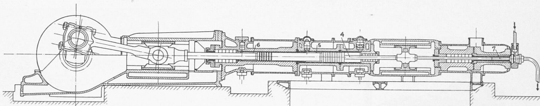
Abb. 3. Schnitt durch den Hochdruckteil (Stufen 4 bis 7) des Burckhardt-Hyperkompressors
