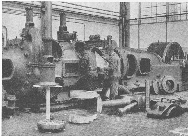
Abb. 2. Niederdruckteil eines Burckhardt-Hyperkompressors
