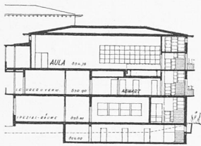
AULA-TRAKT
