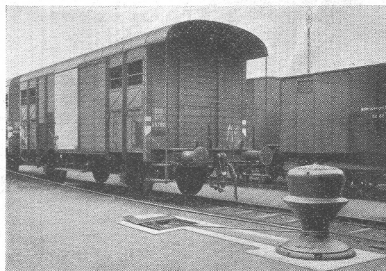
Rangierspilanlage SBB Werkstätte Zürich-Alttetten
