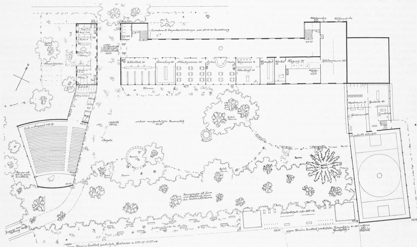
Grundriss des Tiefparterre (424,60). — Masstab 1:600
