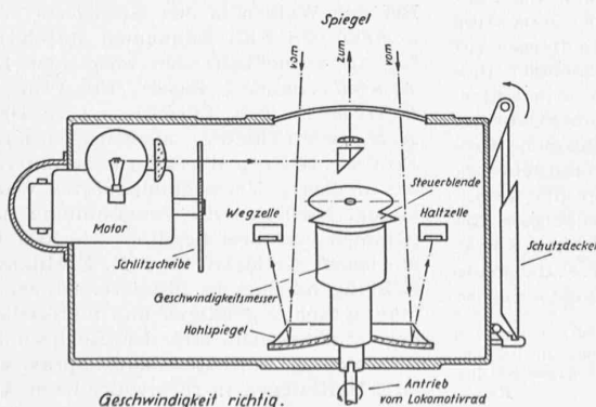
Abb. 3. Tripelspiegel Abb. 4a und b (rechts). Für beliebige Geschwindigkeitsstufen einstellbare Ueberwachung durch Steuerblende am Geschwindigkeitsmesser
