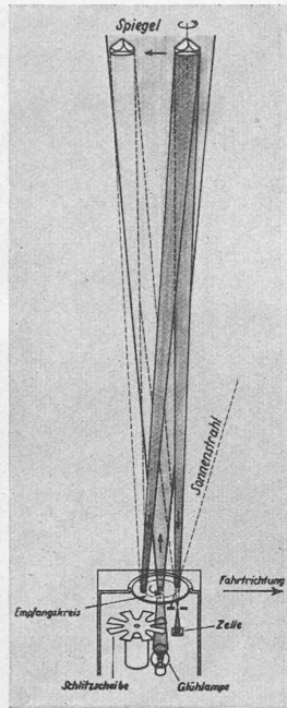
Abb. 2. Wirkungsweise des Tripelspiegels zur optischen Signalübermittlung
