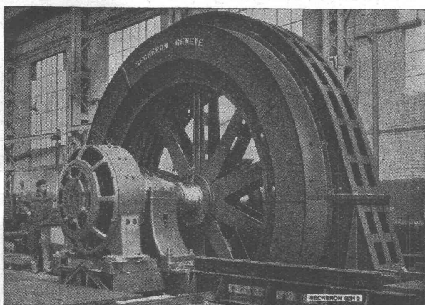
Dreiphasen-Generator von 7000 kVA, 150 t/min in geschweisster Ausführung für ein schwedisches Kraftwerk.
