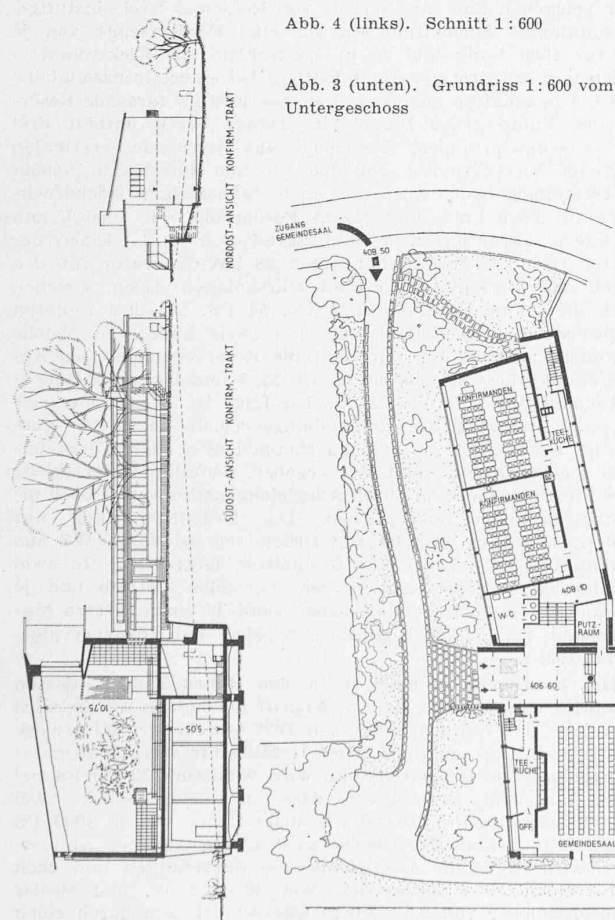
Abb. 4 (links). Schnitt 1:600
