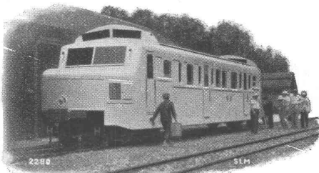
2 x 150 PS Dieselltriebwagen der Yunnan-Bahn (Indochina) ausgerüstet mit „S. L. M.-Winterthur“ Oelschaltgetriebe.
