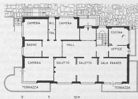
PIANO ABITAZIONE
