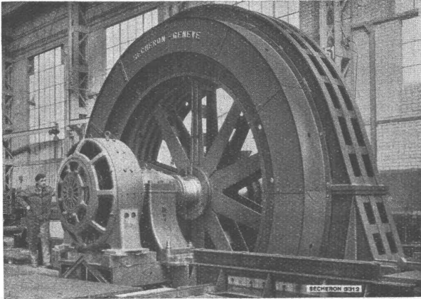
Dreiphasen-Generator von 7000 kVA, 150 t/min in geschweißter Ausführung für ein schwedisches Kraftwerk. Aufstellung im Prüfraum für Abnahmeversuche.
