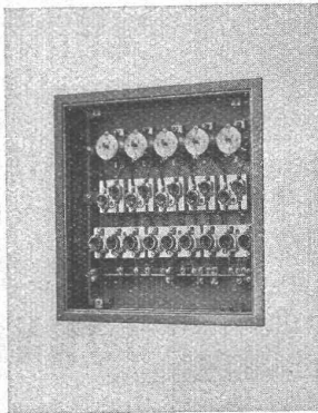
Deckel u. Schutzplatte abgehoben
