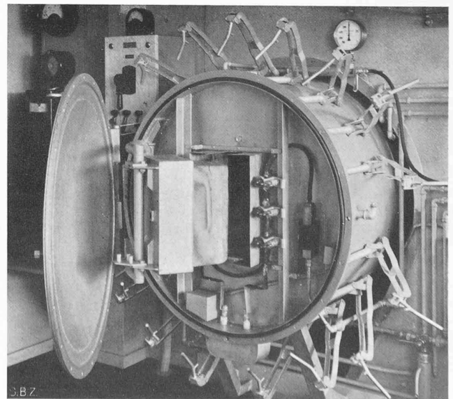
Abb. 4. Muffelöfen für max. 1450°C der Firma Brown, Boveri (Baden)
